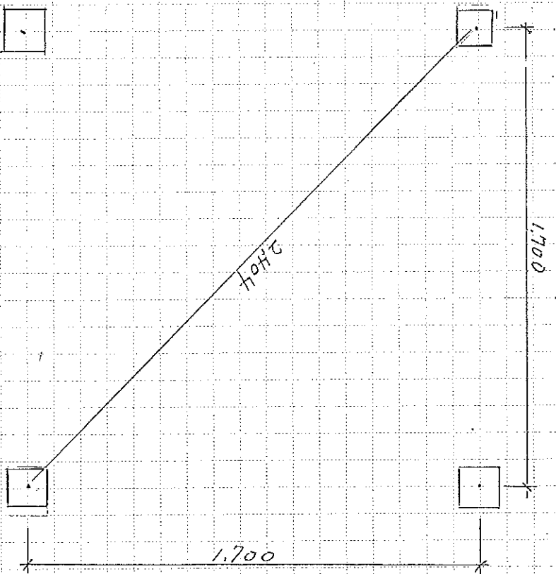
東基礎伏圖
